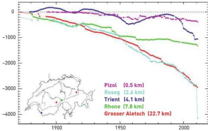
Grafik 3: Längenänderung
